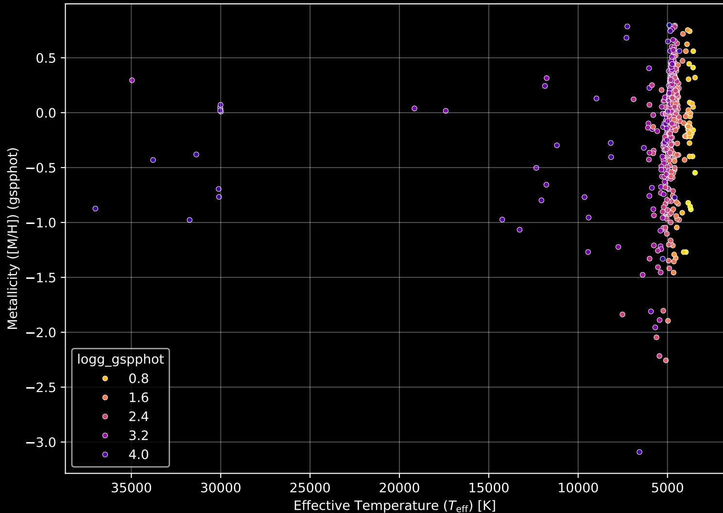
APOGEE DR17 Field: [002-04] Stellar Population Parameters (n= 584)
